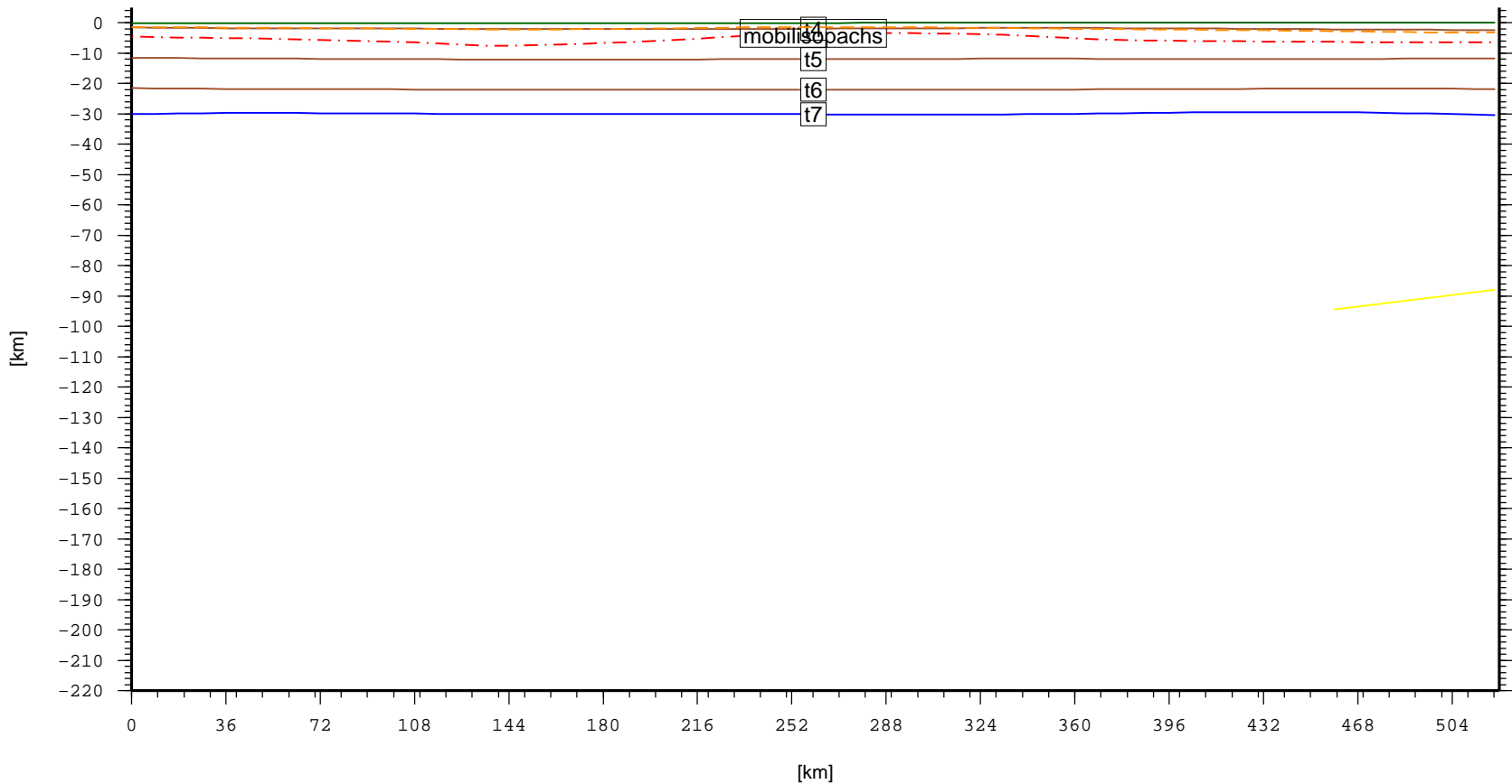
Cross section – EUR.CentralGrabenProvince_NorthSeaGrabenSystem (topo, laske sedthick, t4, t5, t6, t7)
